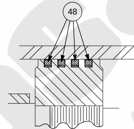
OPTIONAL RING TYPE PISTON
